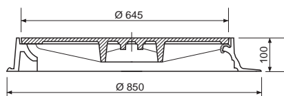
COUPE A-A
