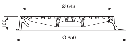
COUPE A-A
